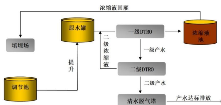
图 1 渗滤液设备处理工艺流程图
